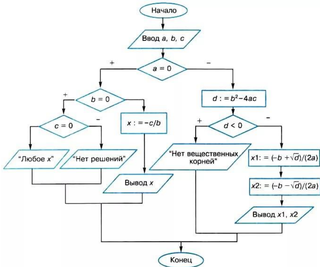
Рис. 3.15. Блок-схема алгоритма решения квадратного уравнения
