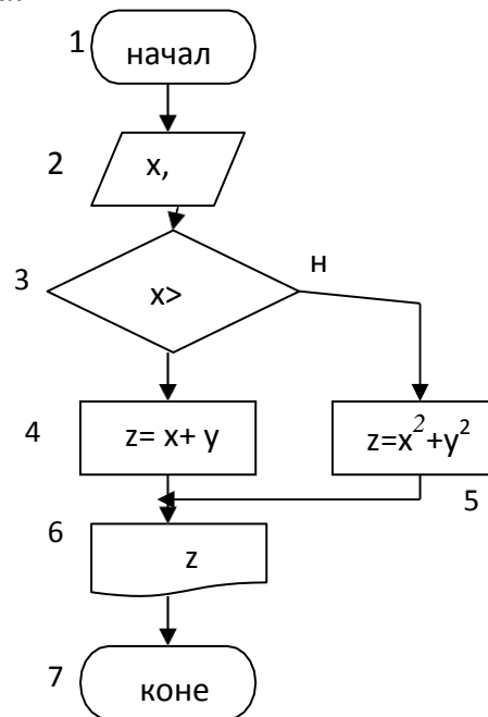
Рис.2. Алгоритм ветвления
