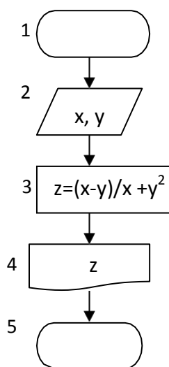
Рис.1. Линейный алгоритм
