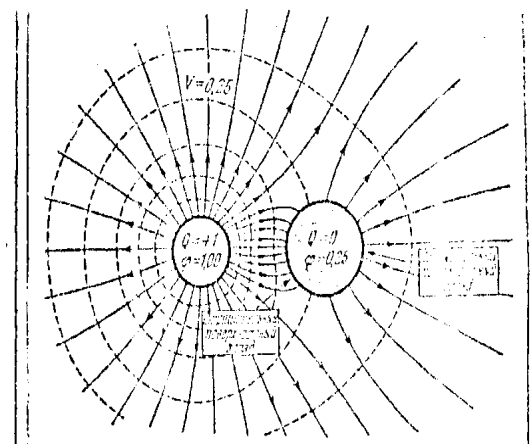
Рис. 3.5. Электрическое поле около двух сферических проводников, из которых один имеет заряд, равный +1, а другой – равный нулю. Пунктирные кривые являются пересечениями эквипотенциальных поверхностей с плоскостью рисунка, Нулевой потенциал находится в бесконечности.
