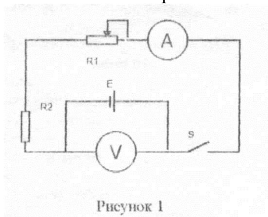
Схема измерений
