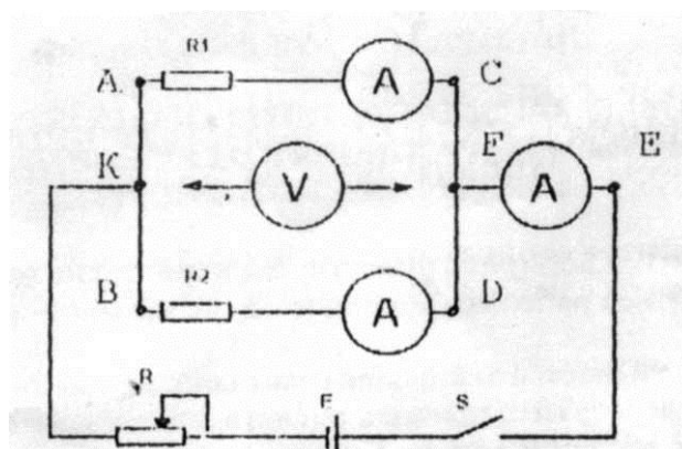
Рисунок 2. Параллельное соединение потребителей
